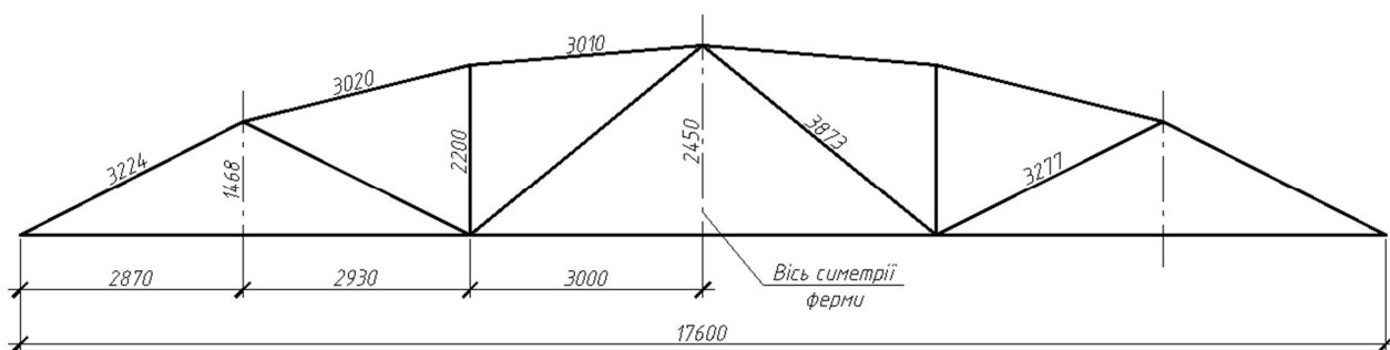
Рис. 2. Геометрична схема ферми
