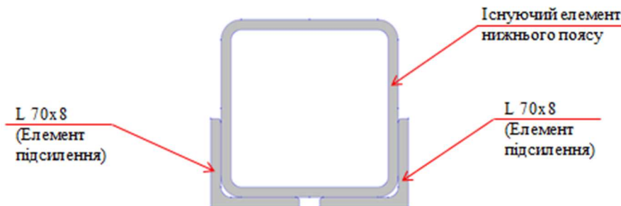
Рис. 3. Схема виконання підсилення
