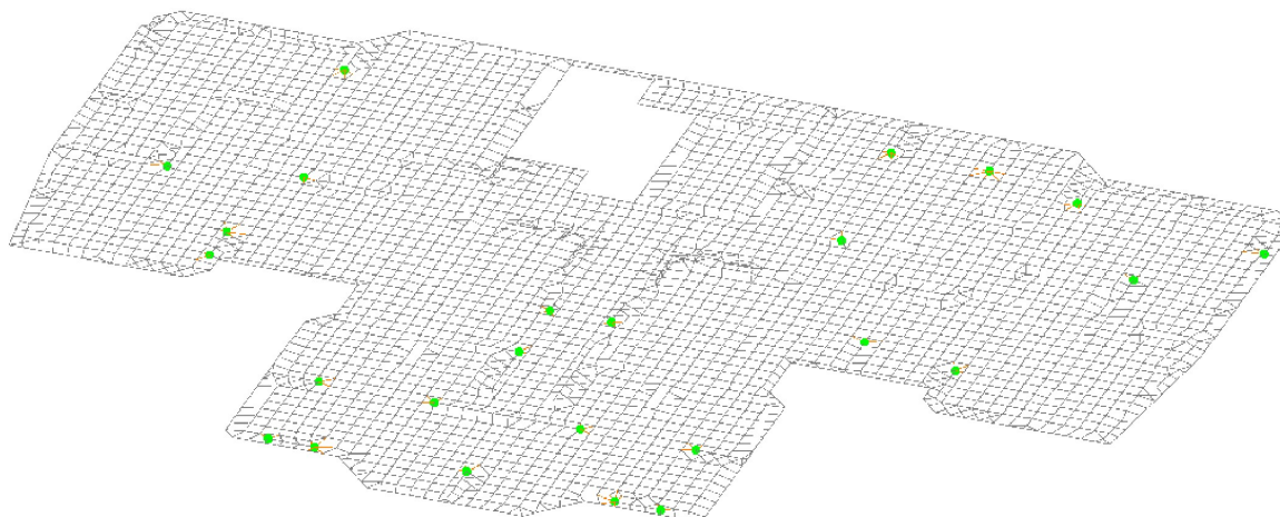
Рис. 1. Розрахункова схема
