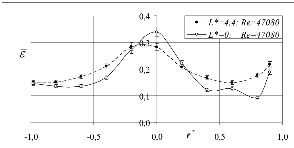
Рис. 3. Профілі відносної інтегральної інтенсивності пульсацій швидкості у вихідному перерізі вихрової камери (довірчі інтервали відносних похибок максимально дорівнюють 4,8% з довірчою ймовірністю 0,9)
