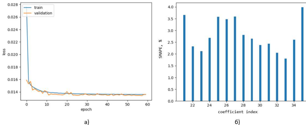
Рис.2. – Результати навчання запропонованої нейронної мережі: а) значення функції втрат протягом навчання; б) середні похибки визначення коефіцієнтів (масштабованих до [0; 1] ) у відсотках.
