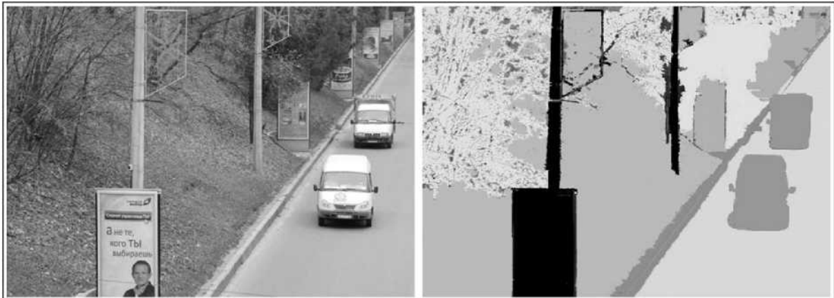
Рисунок 1 – Сегментація відеокадра за допомогою щільної нечіткої кластеризації
