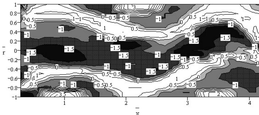
Рис. 1. Приклад розподілу ізотак безрозмірної осьової швидкості в тупиковій частині камери (білий і світло-сірий кольори відповідають напрямку течії праворуч до торця; чорний і темно-сірий кольори – від торця, причому чорний колір відповідає більш високій швидкості), \bar{x} = \frac{x}{d_0}
